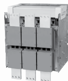
Рис. 6 Выводы для присоединения шин спереди
