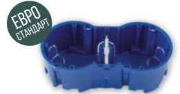
KE-501 Коробка двухместная для крепления выключателей и розеток 136x66x47,4 мм
