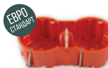
KE-504 Коробка двухместная 136x66x47,4 мм
