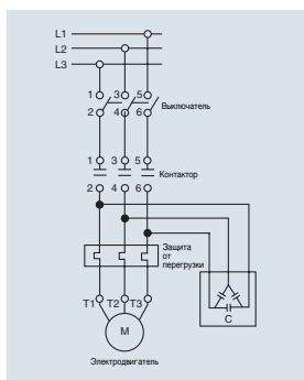
Емкостная цепь
