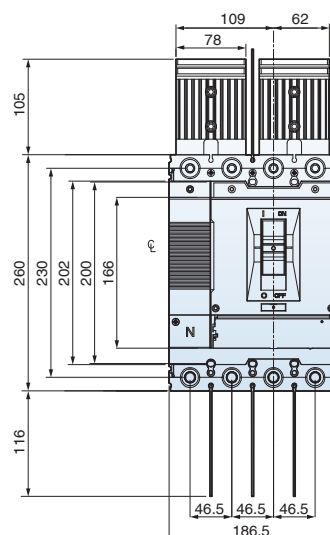
4P (L-типа)
