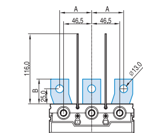
TS400, 630 3P
