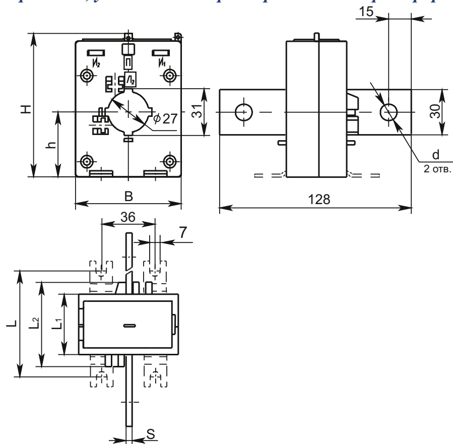
Рис.2 Трансформаторы ТОП на первичные токи 200, 300 и 400 А
