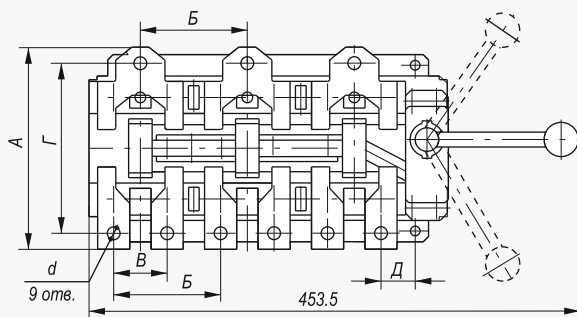
Рисунок 2. Привод правого исполнения.
