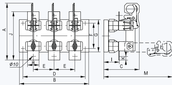
Рисунок 1. Разъединители трехполюсные Р43, Р63
