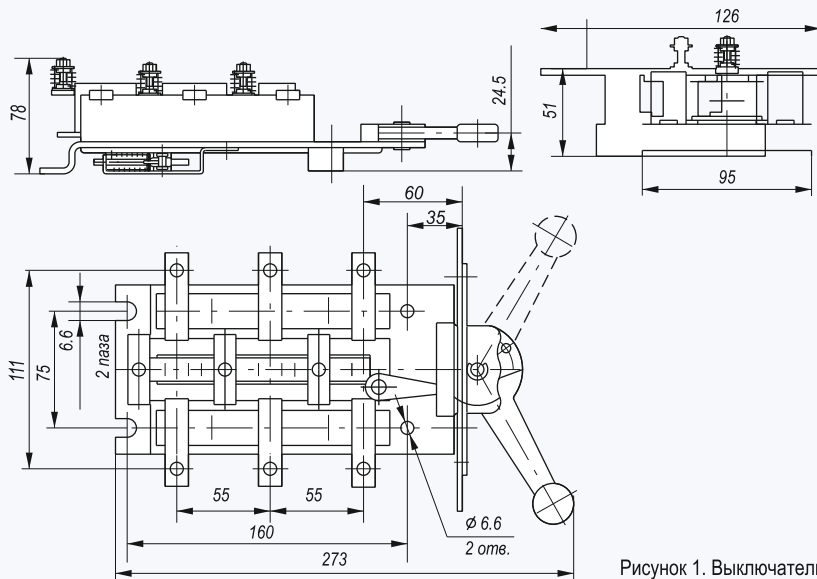
Рисунок 1. Выключатель ВО1-312
