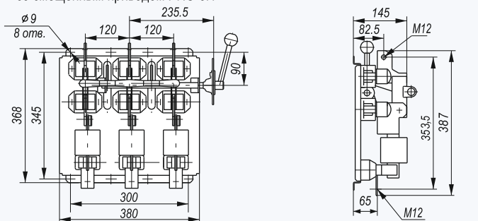
Рисунок 7. Рубильник с предохранителями на общей плите с боковой рукояткой РПБ-6П
