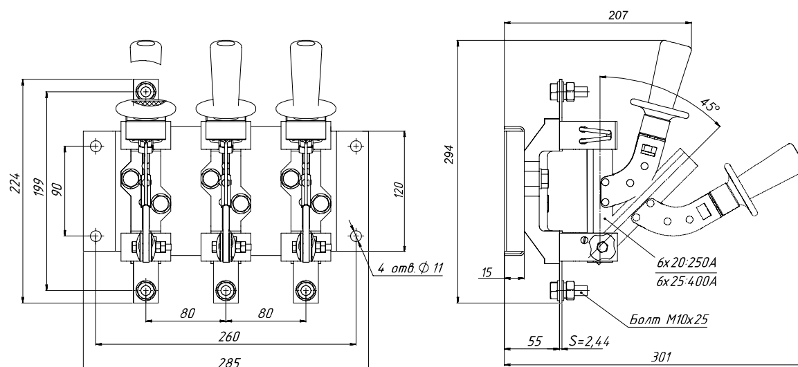
Рис. 5. Разъединитель РЕ19-35(37)-31170-00 УХЛЗ с рукояткой для пополюсного оперирования
