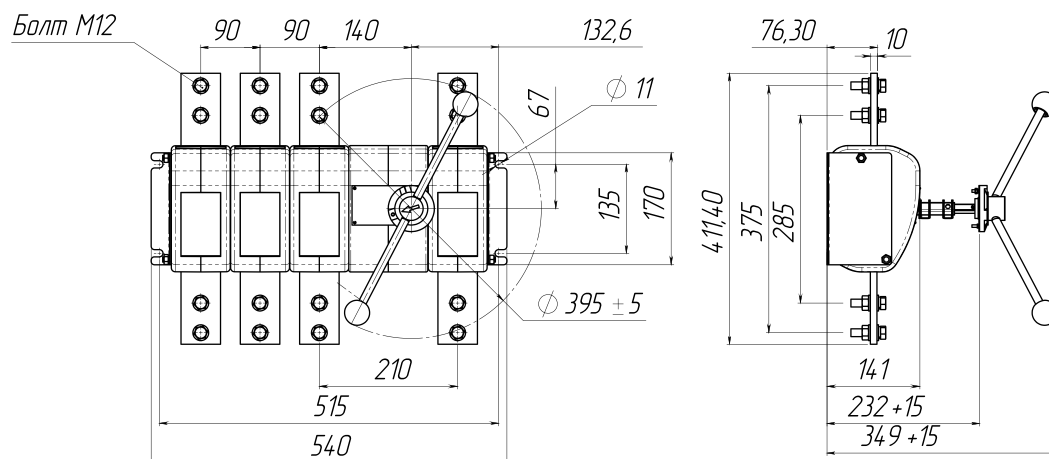
Рис. 7. ВНК-43-41130-32 УХЛ3, масса не более 23,5 кг
