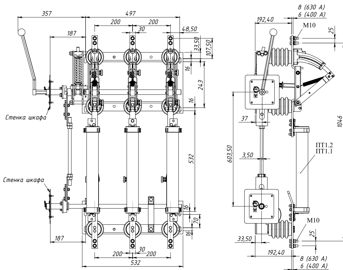
Рис. 20. Выключатель нагрузки автогазовый типа ВНАЛр-10/630-20-IIз ПТ 1.2 (1.1) У2, масса не более 49 кг
