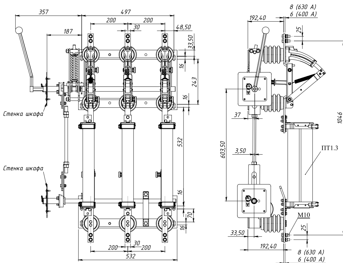
Рис. 21. Выключатель нагрузки автогазовый типа ВНАЛр-10/630-20-IIз ПТ 1.3 У2, масса не более 50 кг
