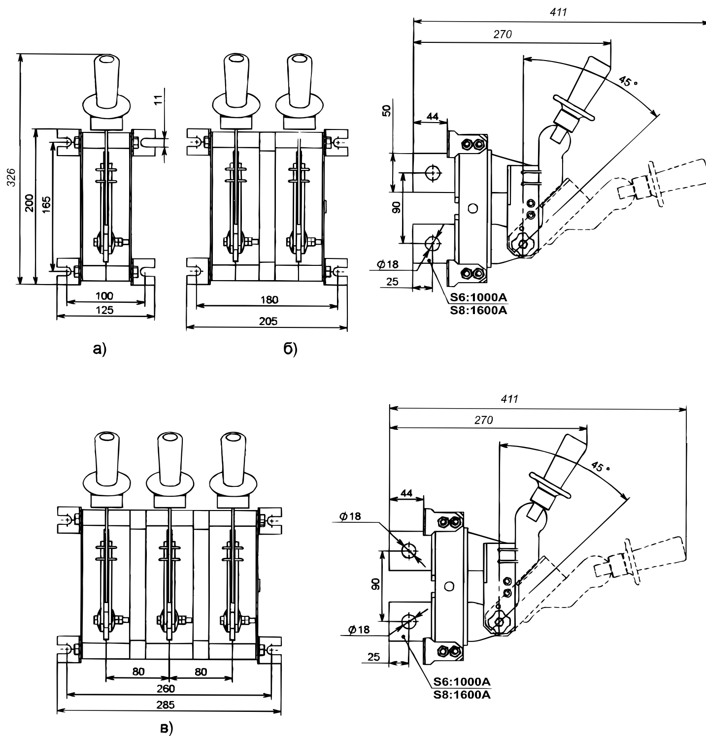
Рис. 28. Разъединитель РЕ19 с рукояткой для пополюсного оперирования, заднего присоединения шин а) РЕ19-41(43)-12270-00 УХЛЗ; б) РЕ19-41(43)-22270-00 УХЛЗ; в) РЕ19-41(43)-32270-00 УХЛЗ
