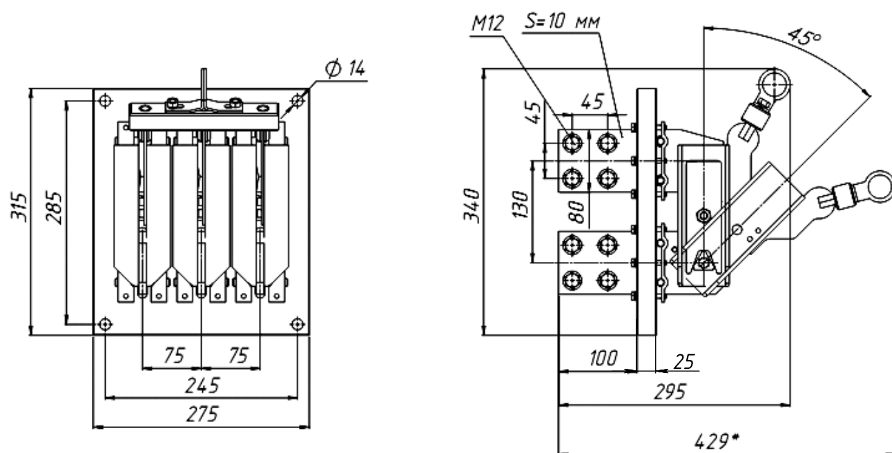
Рис. 56. Разъединитель PE19 с центральным рычагом для управления штангой, на изоляционной плите PE19-49-12290-00 УХЛ3, и/п
