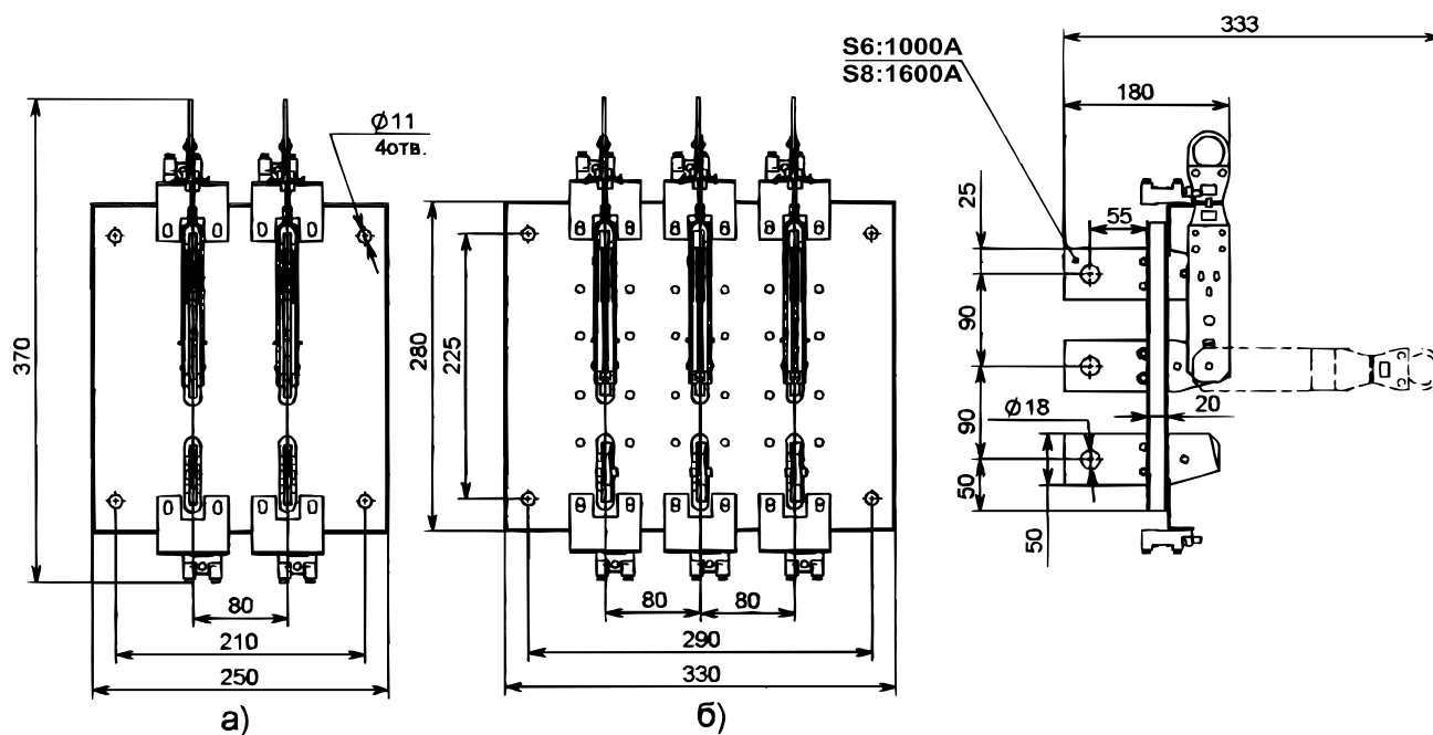
Рис. 41. Разъединитель PE19 на два направления с рукояткой для полюсного оперирования, на изоляционной плите а) PE19-41(43)-62271-00 УХЛЗ, и/п; б) PE19-41(43)-72271-00 УХЛЗ, и/п
