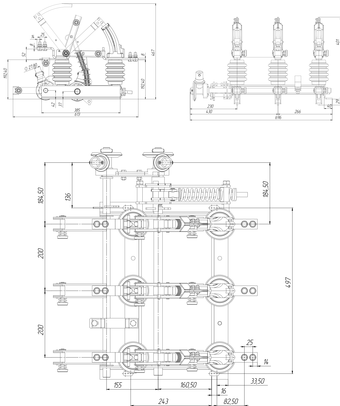
Рис. 25. Выключатель нагрузки автогазовый типа ВНАЛш-10/630-20-ІІзУ2, масса не более 38 кг
