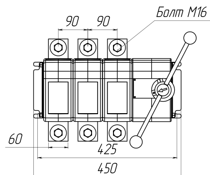
Рис. 10. ВНК-41-31130-32 УХЛ3, масса не более 17,5 кг
