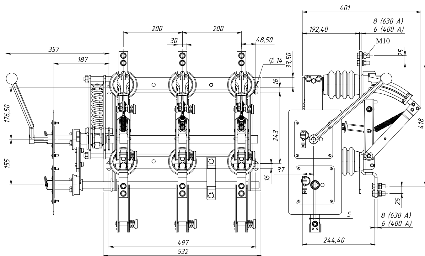
Рис.15. Выключатель нагрузки автогазовый типа ВНАЛр-10/630-20-IIIз У2, масса не более 38,3 кг
