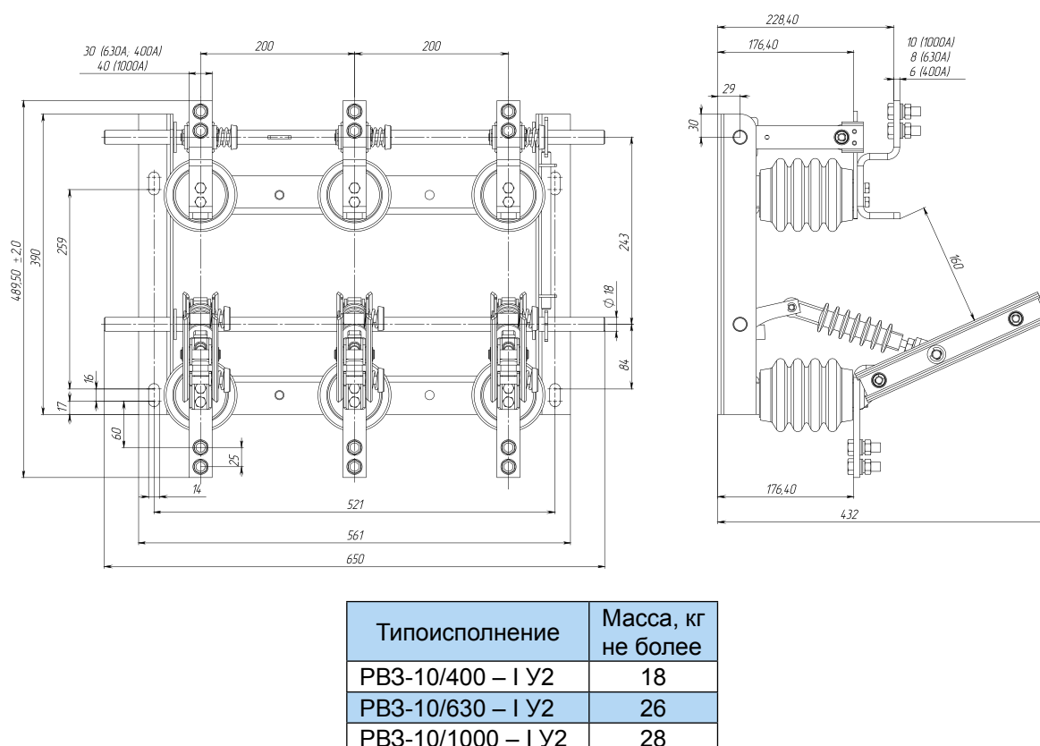
Рис. 2. Разъединитель внутренней установки типа PB3, заземляющие ножи со стороны разъёмных контактов
