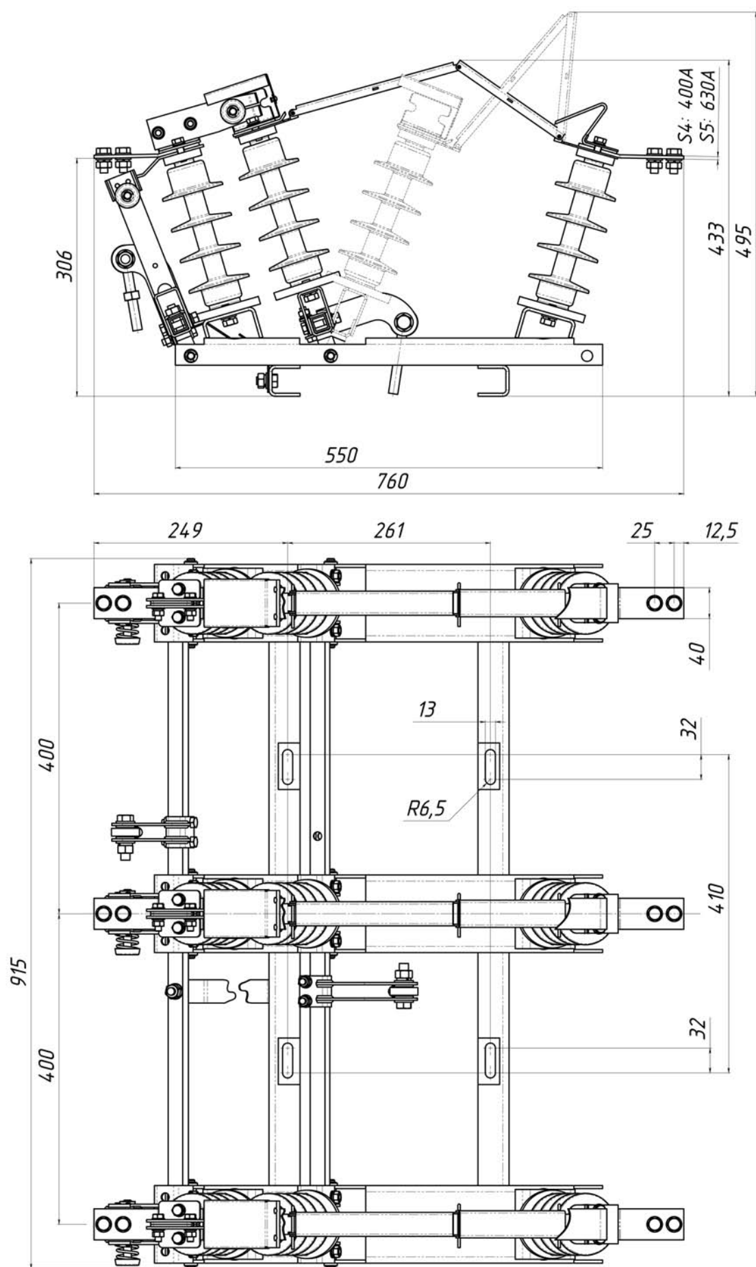
Рис. 2. Разъединитель РЛК-1а-II-10/400(630) УХЛ1, масса не более 42,2 (43,7) кг
