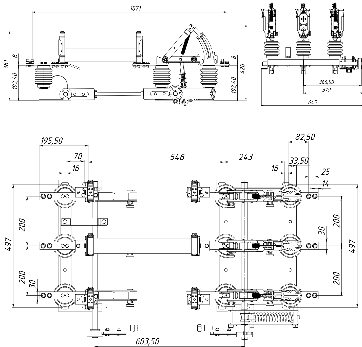
Рис. 5. Выключатель нагрузки автогазовый типа ВНАП-10/630-20-IIз ПТ 1.3 У2, масса не более 47 кг
