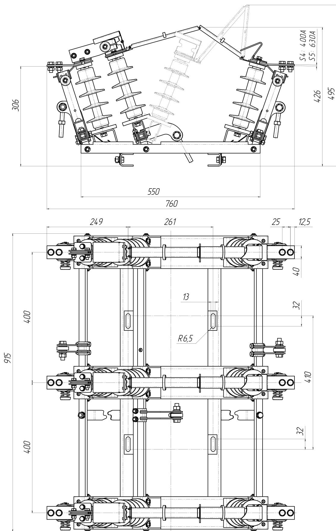
Рис. 1. Разъединитель РЛК-2-II-10/400(630) УХЛ1, масса не более 46,8 (48,3) кг
