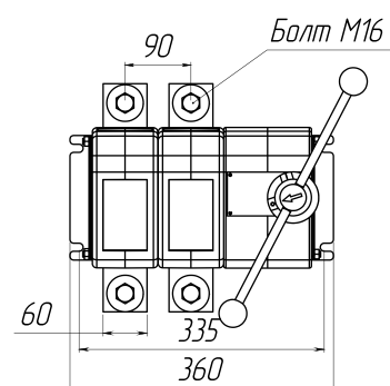
Рис. 12. ВНК-41-21130-32 УХЛ3, масса не более 13,2 кг
