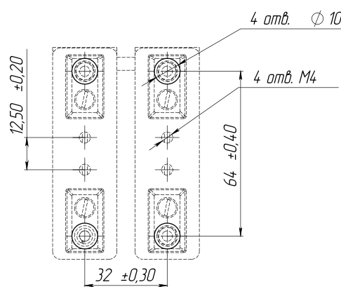
Разметка панели под установку комплекта из двух Р-25-1121
