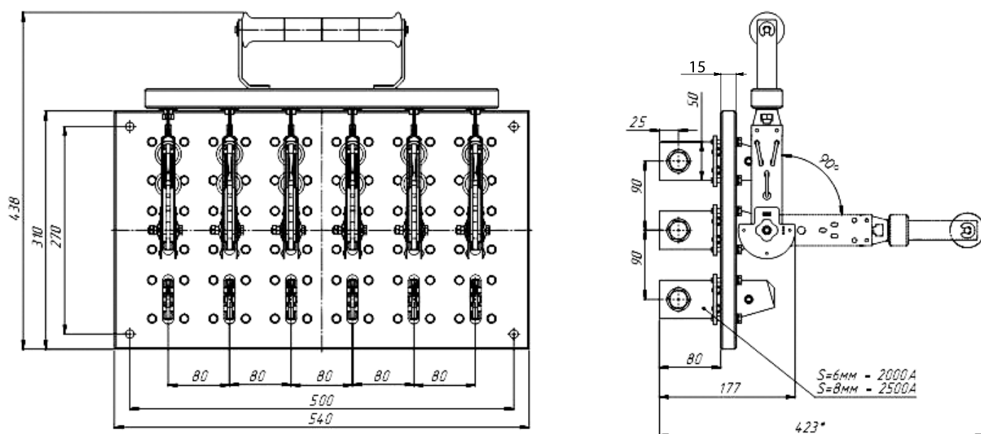
Рис. 55. Разъединитель PE19 на два направления с центральной рукояткой, на изоляционной плите PE19-44(45, 46)-72210-00 УХЛ3, и/п
