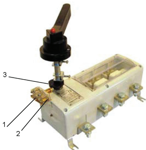
Рис. 1. Выключатель-разъединитель ВНК на токи 250 А, 400 А и 630 А
