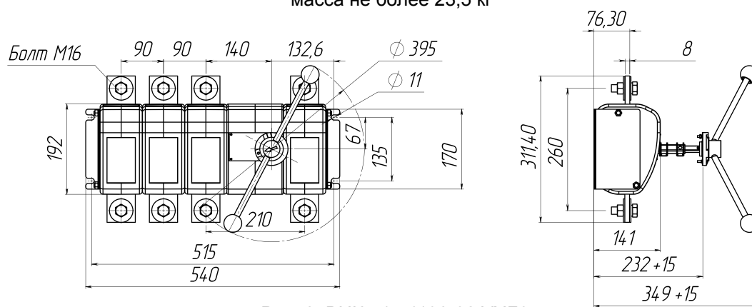
Рис. 8. ВНК-41-41130-32 УХЛ3, масса не более 21,8 кг
