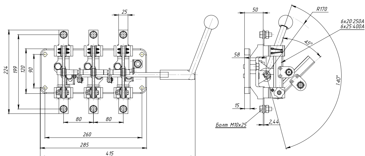
Рис. 6. Разъединитель РЕ19-35(37)-31150-00 УХЛЗ с боковой смещенной рукояткой
