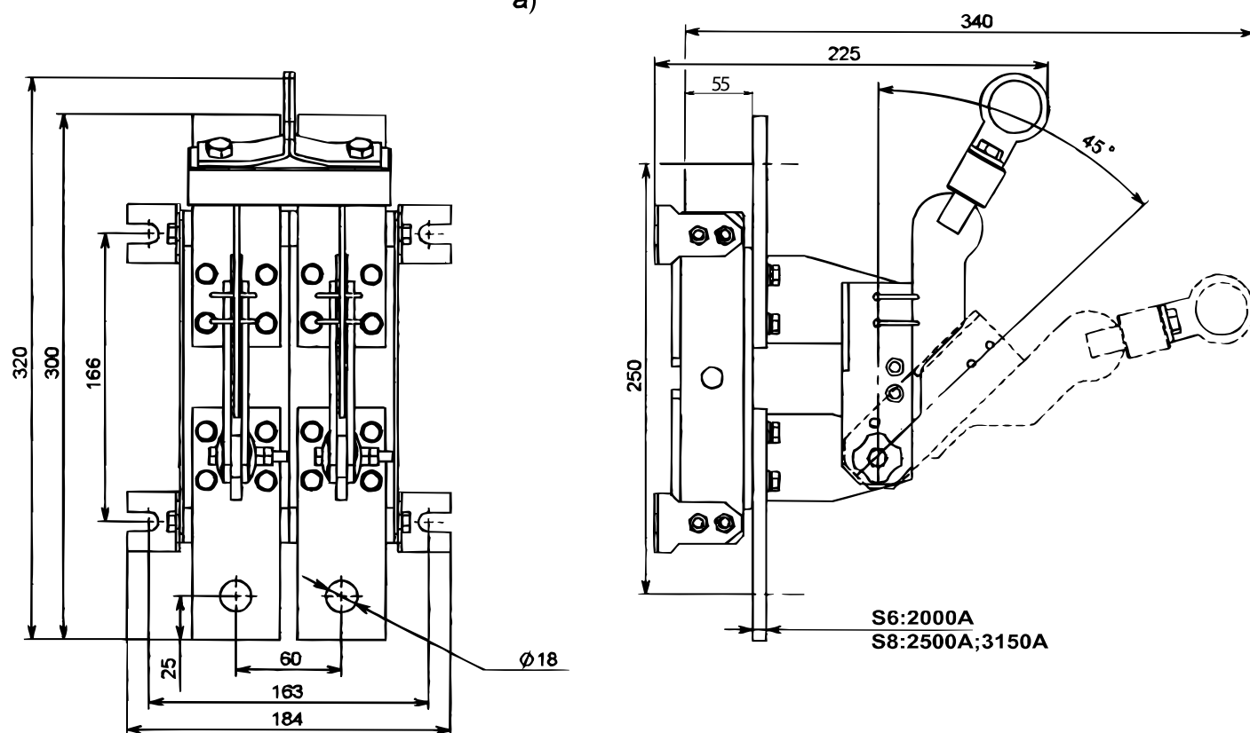
Рис. 45. Разъединитель РЕ19 однополюсный а) РЕ19-44(45; 46)-11110-00 УХЛЗ с центральной рукояткой; б) РЕ19-44(45; 46)-11190-00 УХЛЗ с центральным рычагом для управления штангой
