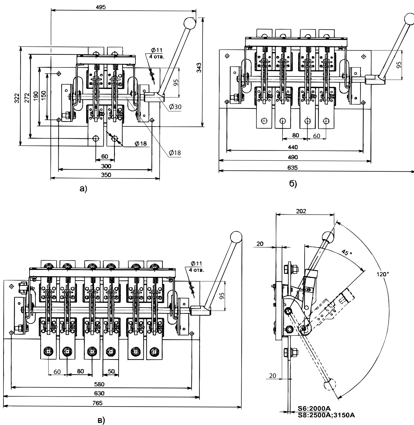
Рис. 51. Разъединитель РЕ19 с боковой рукояткой, на изоляционной плите а) РЕ19-44(45, 46)-11120-00 УХЛЗ, и/п; б) РЕ19-44(45, 46)-21120-00 УХЛЗ, и/п; в) РЕ19-44(45, 46)-31120-00 УХЛЗ, и/п
