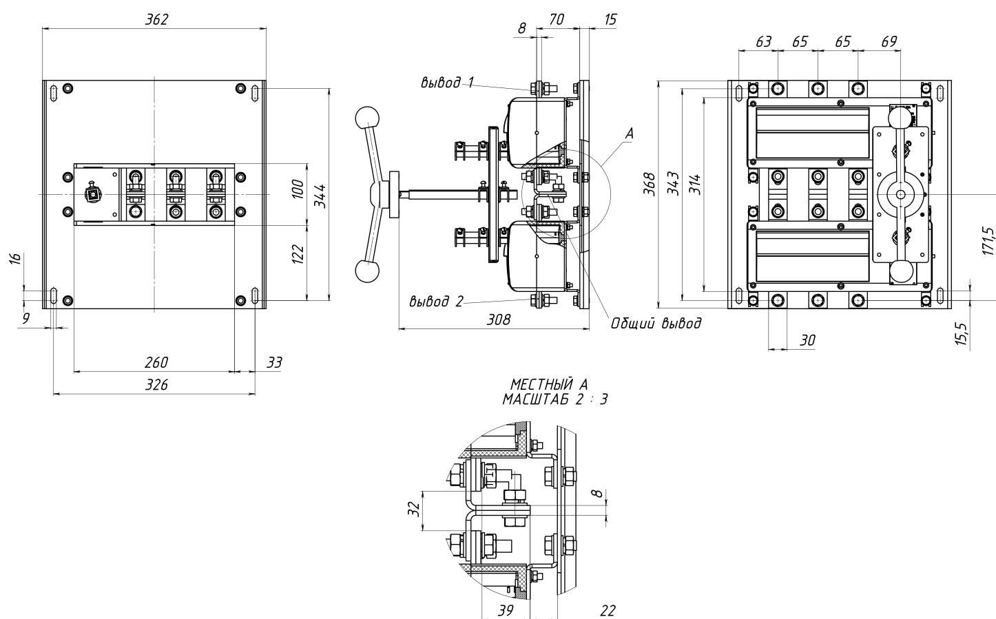
Рис. 4. Выключатель-разъединитель ВНК-37-71130-32 УХЛ3 на два направления, масса не более 12,5 кг
