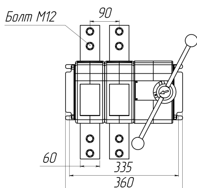
Рис. 11. ВНК-43-21130-32 УХЛ3, масса не более 14,1 кг
