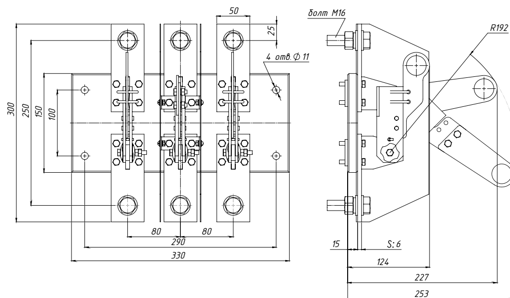
Рис.11. Разъединитель Р103 с пополюсным оперированием штангой ШО-1, на номинальный ток 1000 А
