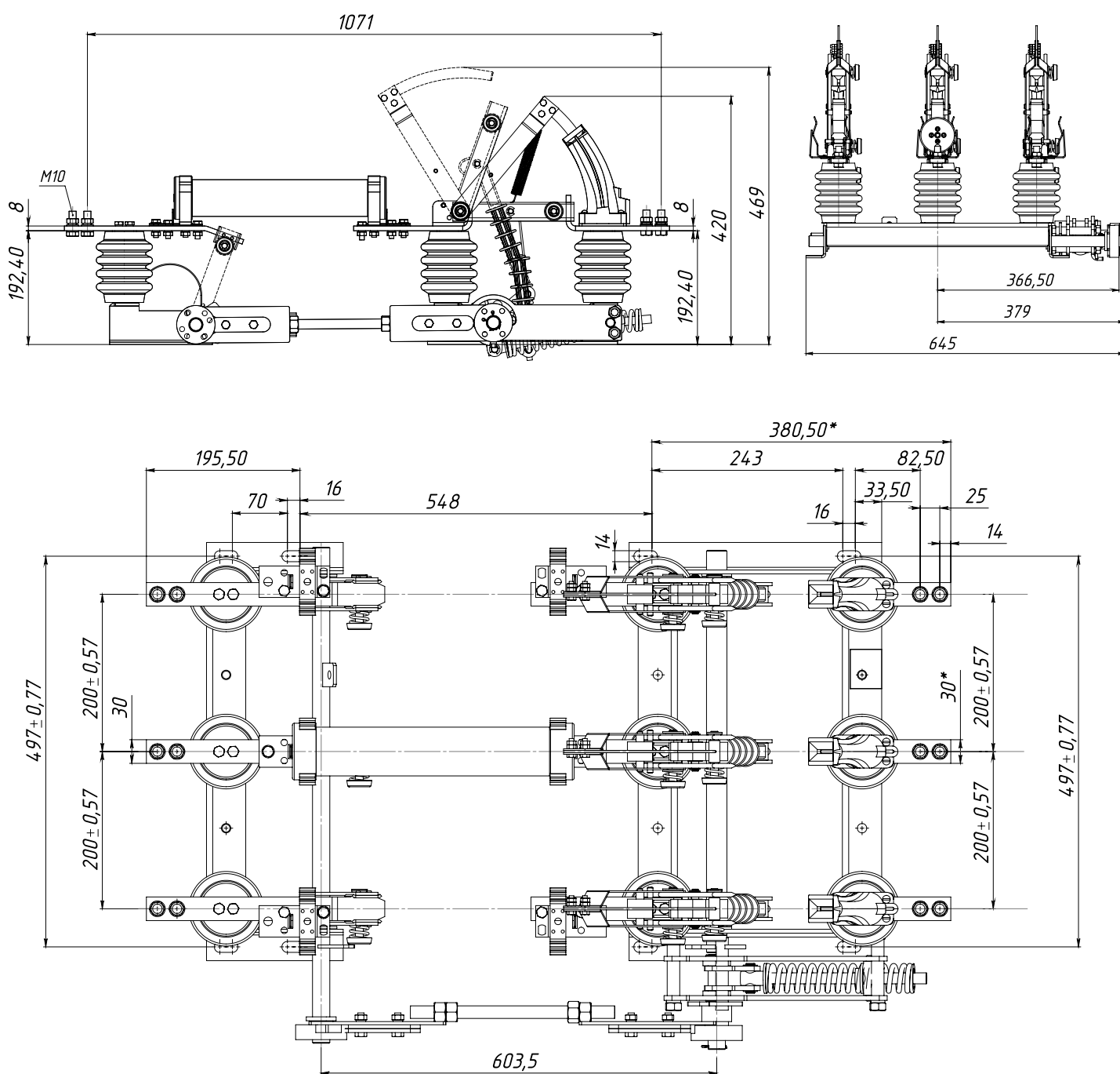
Рис. 3. Выключатель нагрузки автогазовый типа ВНАП-10/630-20-IIIз ПТ 1.2 У2, масса не более 46,5 кг
