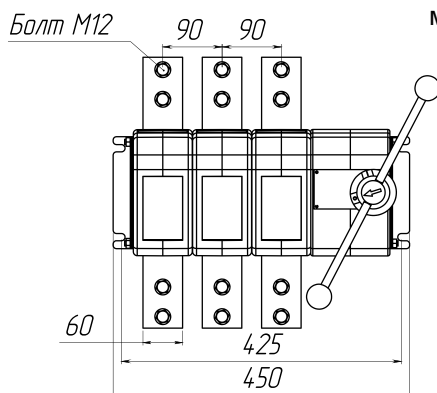
Рис. 9. ВНК-43-31130-32 УХЛ3, масса не более 18,8 кг
